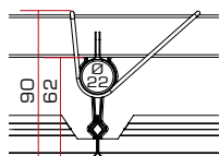
A. SMUSSATO - BEVELLED EDGE
