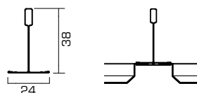
24 LINEAR TEGULAR ribassati di 8/15 mm 8/15 mm lowered
