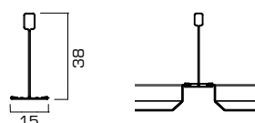
15 LINEAR DESIGN ribassati di 8/15 mm 8/15 mm lowered
