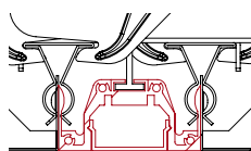
SEZIONE PANNELLO STANDARD 600x600 mm STANDARD TILE'S SECTION
