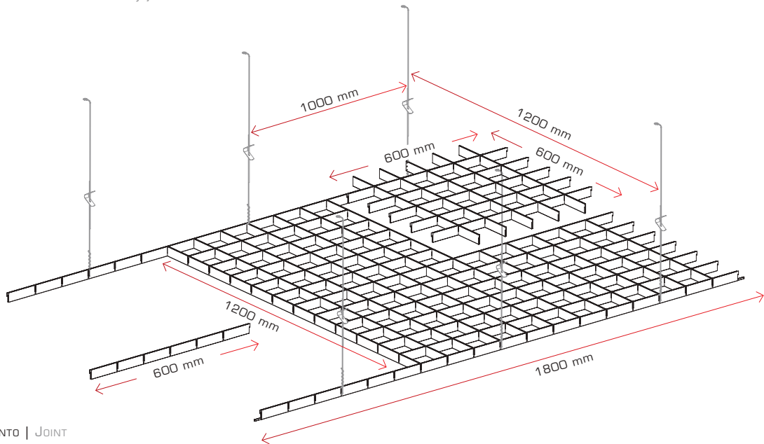
GIUNTO | JOINT
