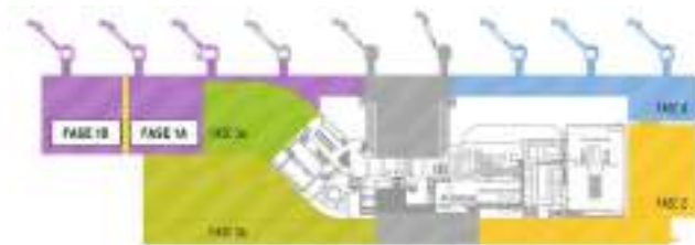
Fasi di ampliamento del terminal passeggeri individuate dal progetto preliminare approvato da Eiras
