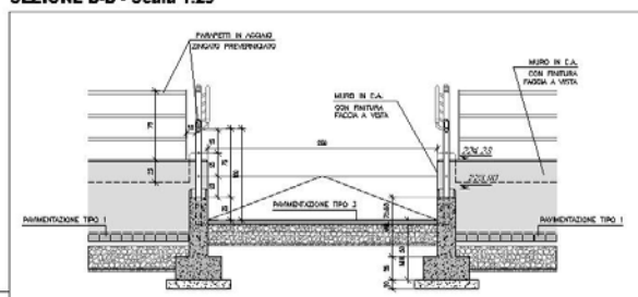
SEZIONE B-B - Scala 1:25
